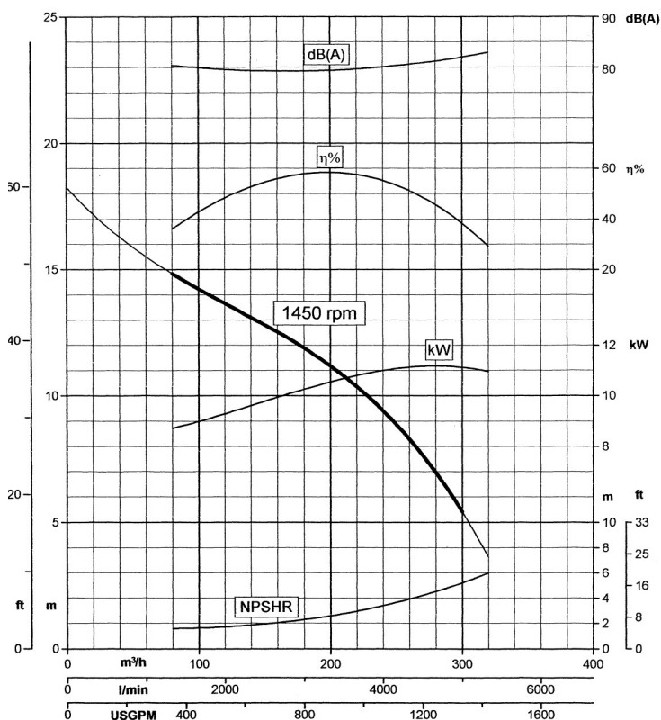
Curva con motore a 1450 rpm
