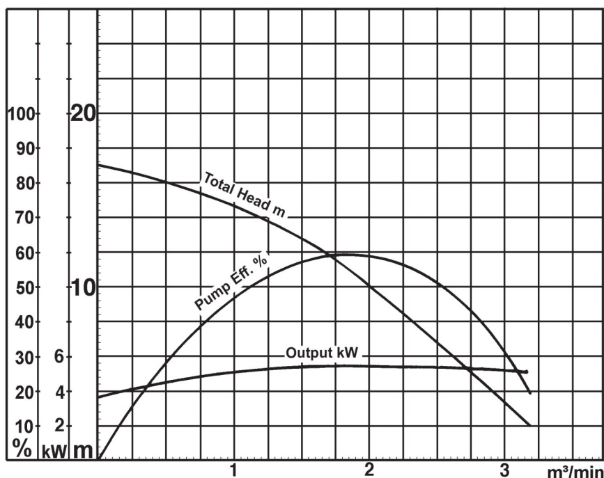
Curva con motore a 1450 rpm
