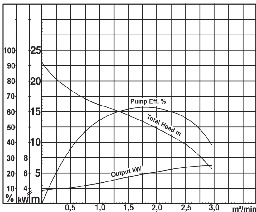
Curva con motore a 1450 rpm
