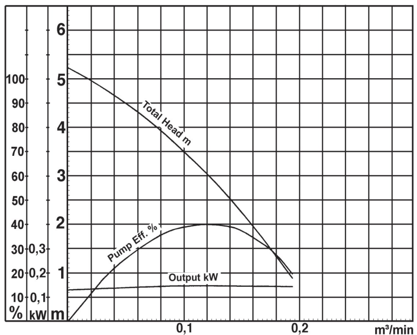
Curva con motore a 2900 rpm
