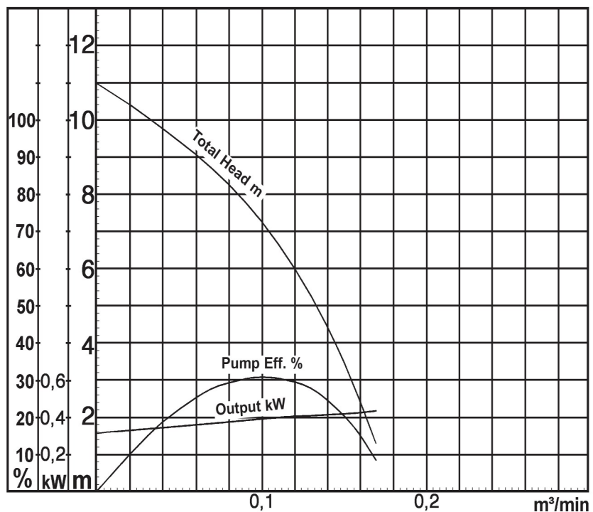
Curva con motore a 2900 rpm
